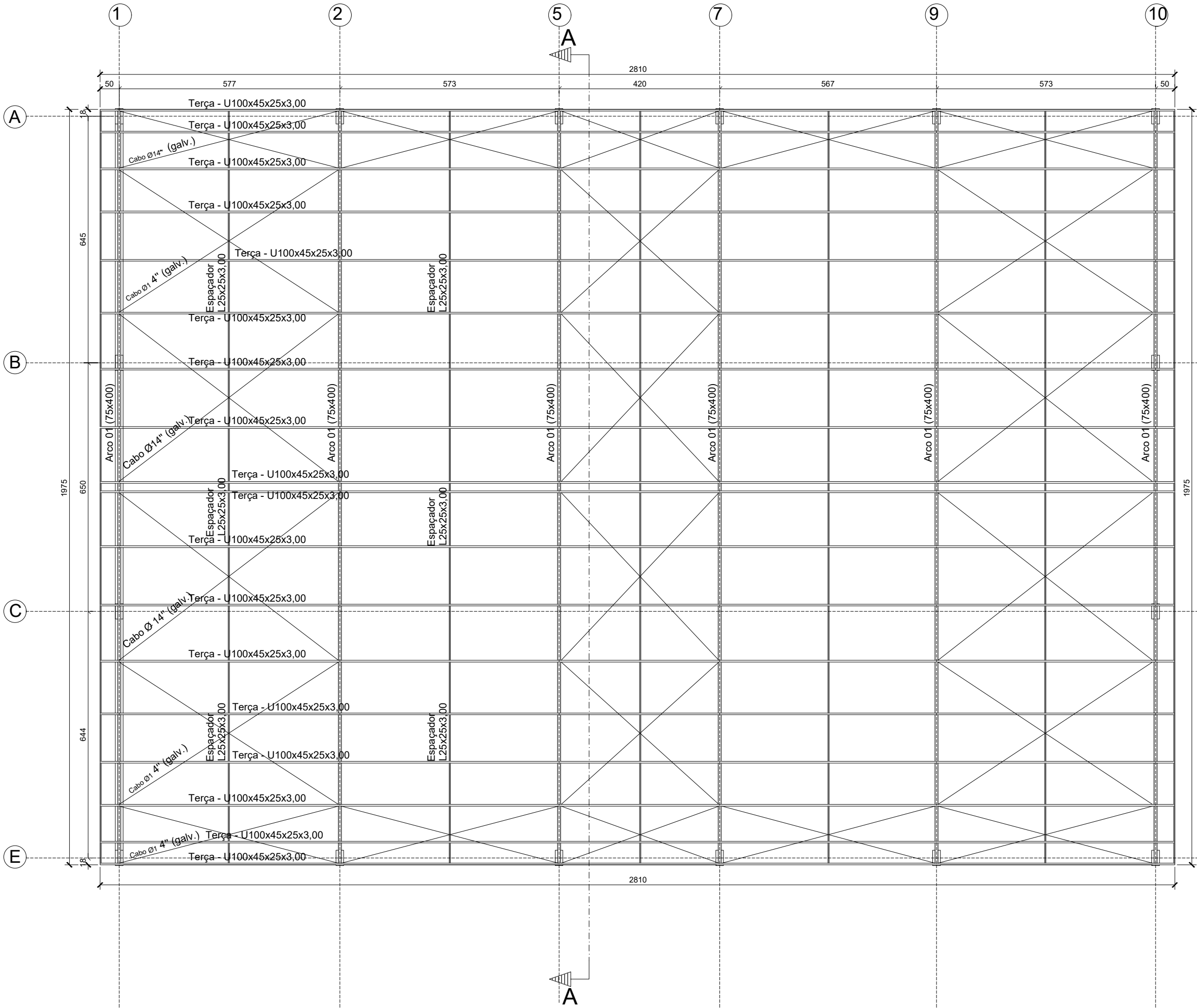
PLANTA ESTRUTURA DE COBERTA (GINÁSIO) (Escala 1:50)
